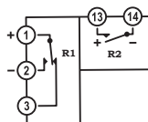
NO/NC Contact*
