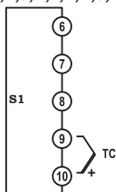
TC Inputs (B,E,J,K,L,N,R,S,T,U)
